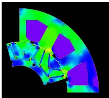
モータ電磁場解析
